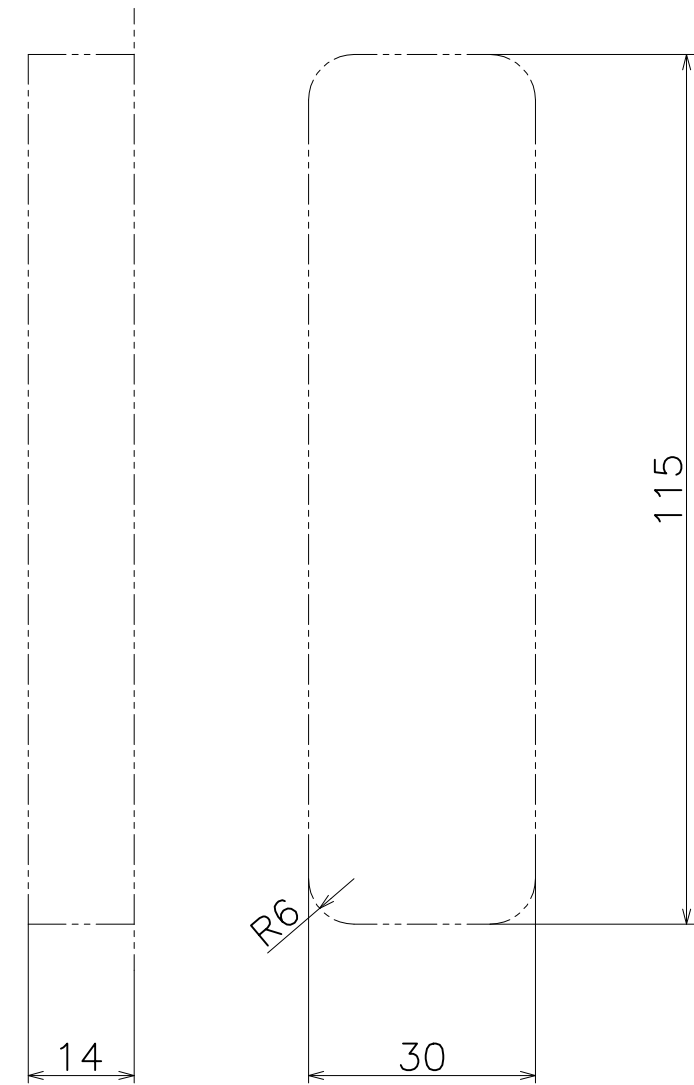
切欠図 (S=1:1)
